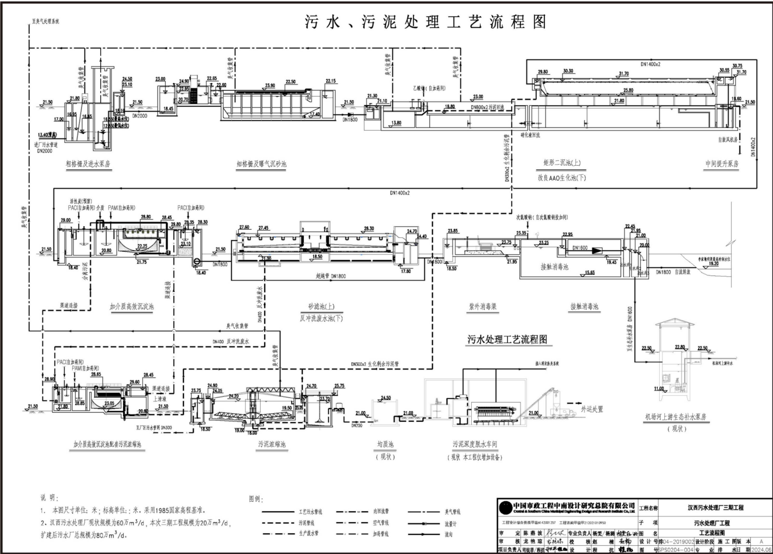
附图 5 三期工程处理工艺流程图
