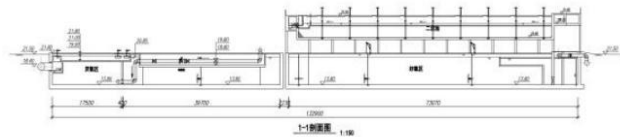
生化池和二沉淀叠放剖面图
