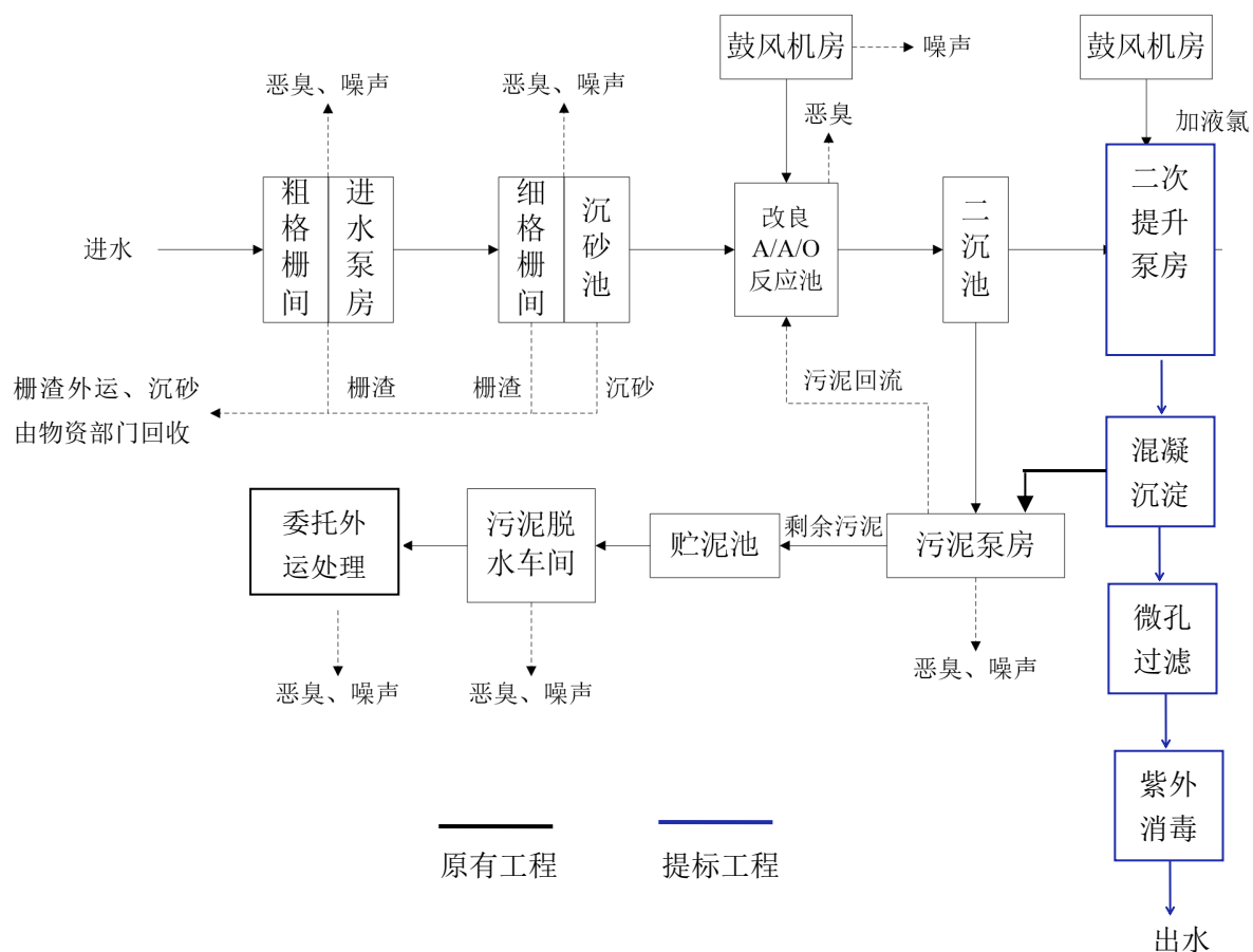
图 3-3 提标工程工艺流程及产污节点图
