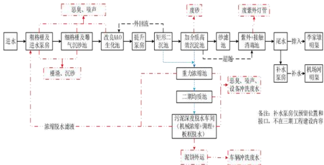
图 3-4 三期工程污水污泥处理工艺流程示意图
